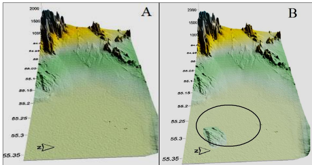
شکل ۷: شکل A صحنه کوهستان و گلاسی قبل از وقوع پدیده بالاآمدگی نشان داده شده و شکل B تغییر در فرم دشت
