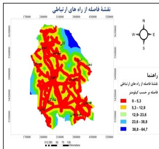
شکل ۷: نقشه فاصله و نقشه استاندارد سازی شده برای معیار فاصله از راه های ارتباطی
