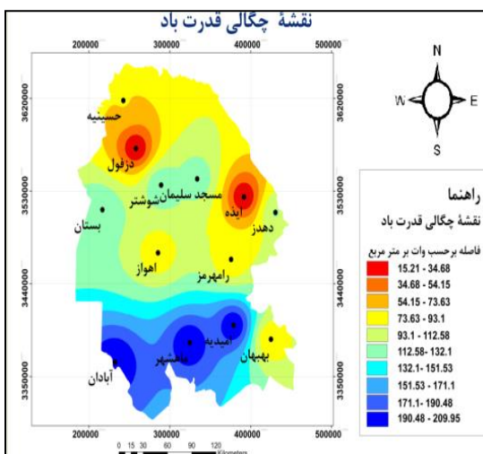
شکل ۱۱: نقشه فاصله و نقشه استاندارد سازی شده برای معیار چگالی قدرت باد
