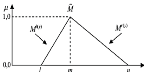
شکل ۱: تابع عضویت عدد مثلثی فازی ( \tilde{M} ) (منبع: (Daneshvar Rouyendegh and Erkan, 2012:924)
