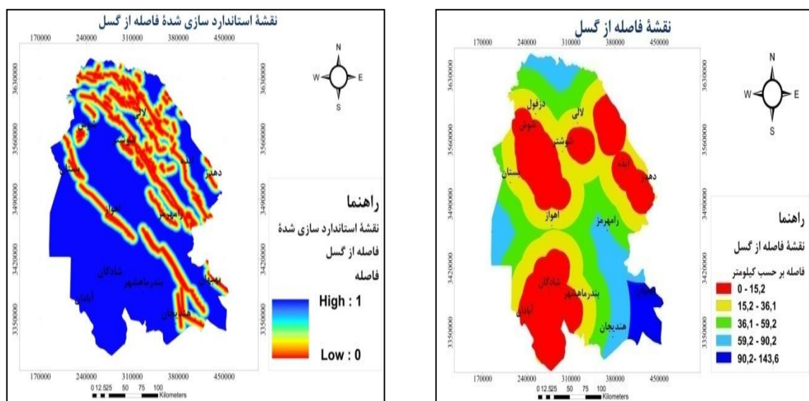
شکل ۱۳: نقشه فاصله و نقشه استاندارد سازی شده برای معیار فاصله از گسل
