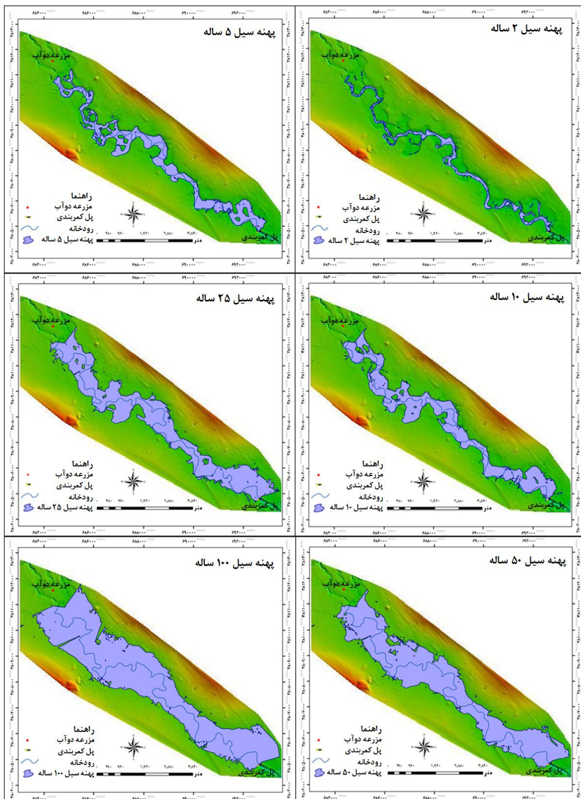
شکل ۵: نقشه پهنه های سیل در دوره بازگشت های مختلف
