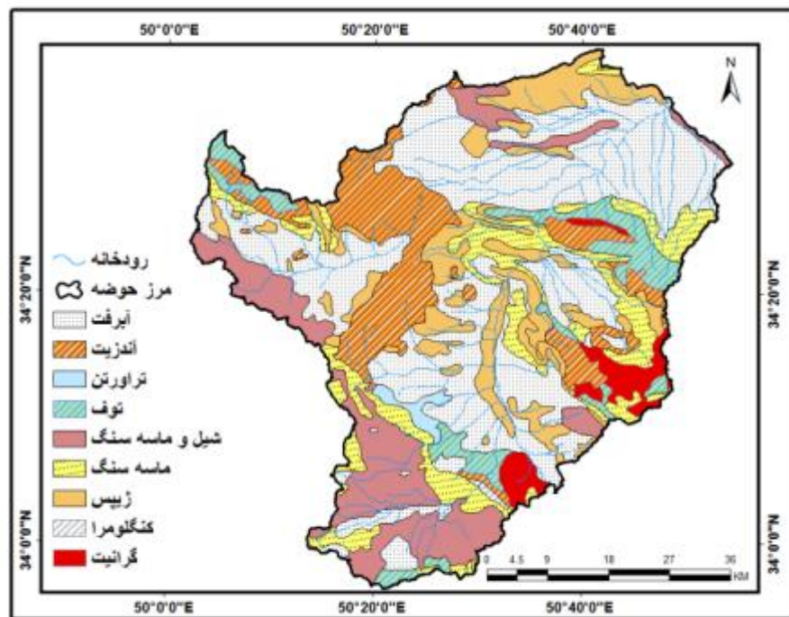
شکل ۷: نقشه لیتولوژی حوضه آبخیز قمرود
