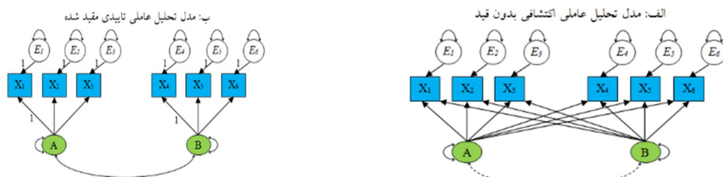
شکل ۲: یک مدل تحلیل عاملی اکتشافی و یک مدل عاملی تاییدی برای ۶ شاخص و ۲ عامل
