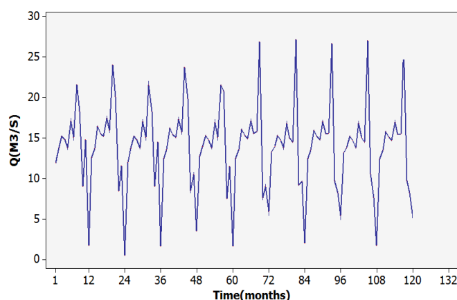
شکل ۱۲: نمودار حاصل از پیش‌بینی مدل ARIMA(1,1,1)(2,0,2) (۲،۰،۲) (۱۰ سال آینده)
