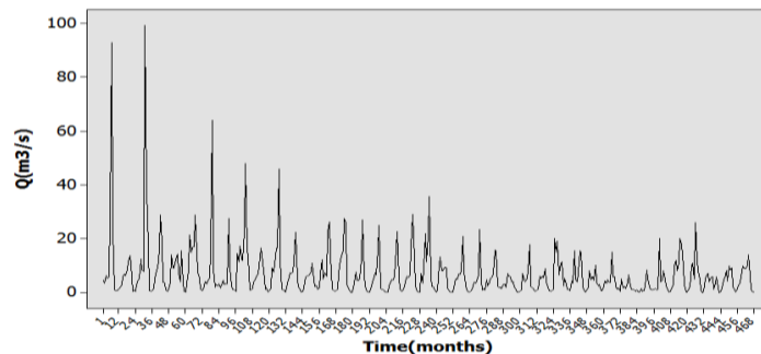
شکل ۸: سری زمانی دبی متوسط ماهانه رودخانه مهران رود (۱۳۹۸-۱۳۵۸)
