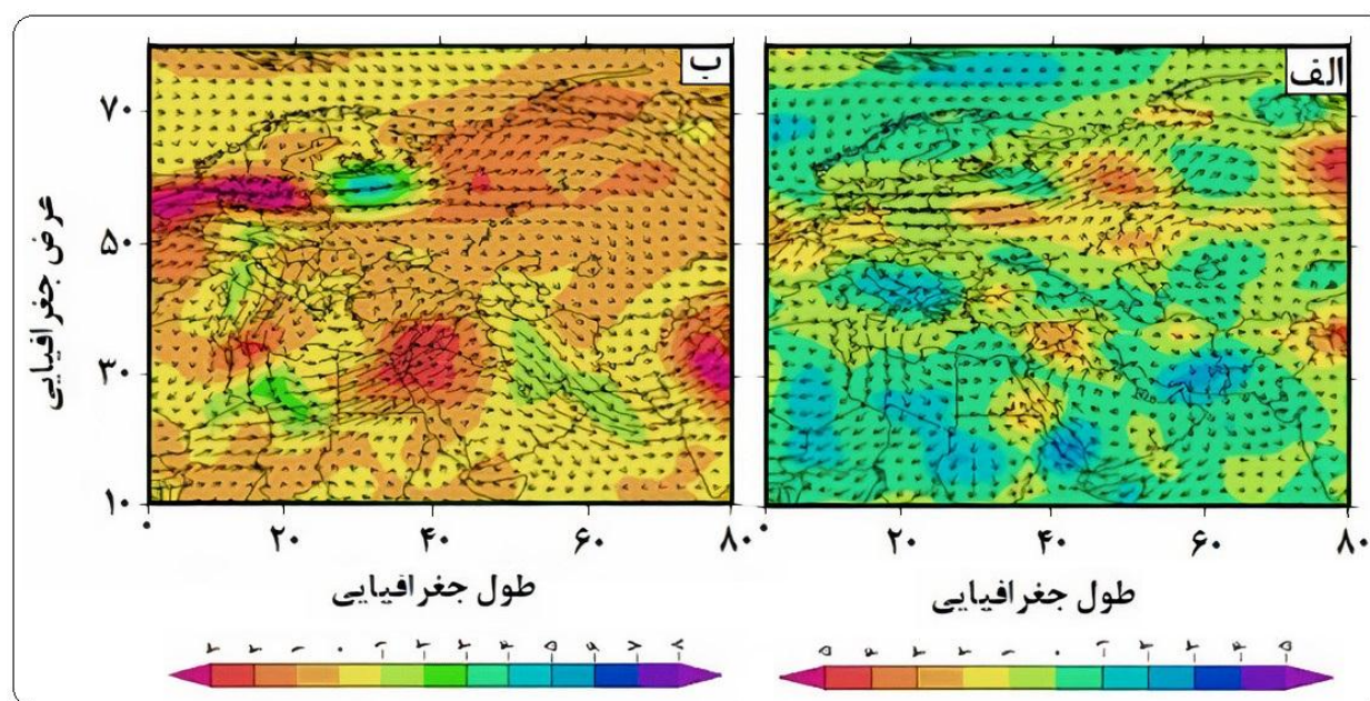
شکل ۱۱: فرارفت دما و جهت جریان های هوا در ترازهای ۸۵۰ (الف) و ۵۰۰ (ب) هکتوپاسکال برای الگوی پنجم
