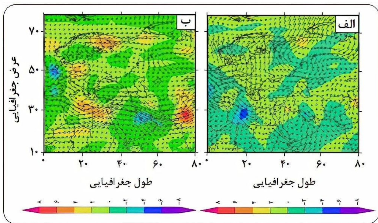
شکل ۷: فرافت دما و جهت جریان‌های هوا در ترازهای ۸۵۰ (الف) و ۵۰۰ (ب) هکتوپاسکال برای الگوی سوم
