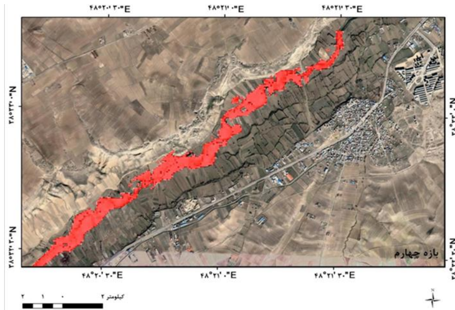
شکل ۷: پهنه‌های سیلابی رودخانه بالیخلی‌چای در بازه چهارم با دوره بازگشت‌های مختلف
