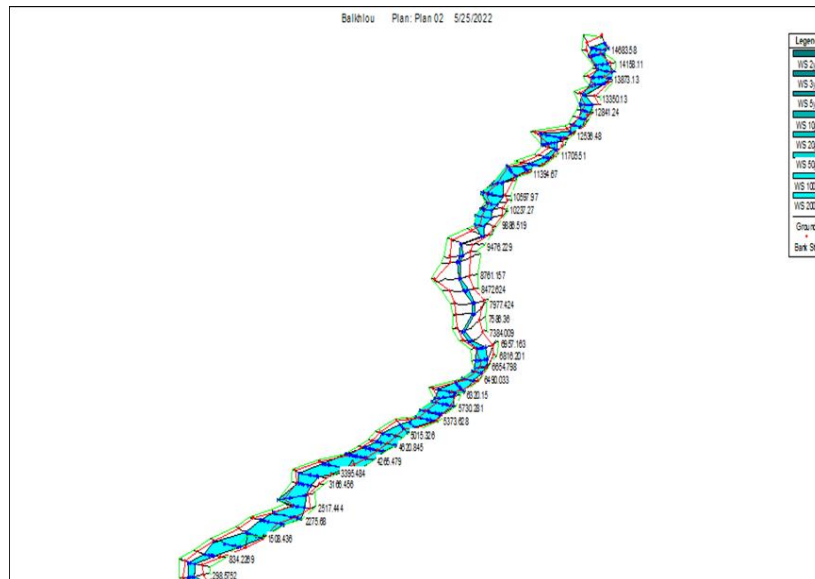
شکل ۸: شبیه‌سازی سیلاب رودخانه بالیخلی‌چای با دوره بازگشت‌های مختلف در نرم‌افزار HEC-RAS
