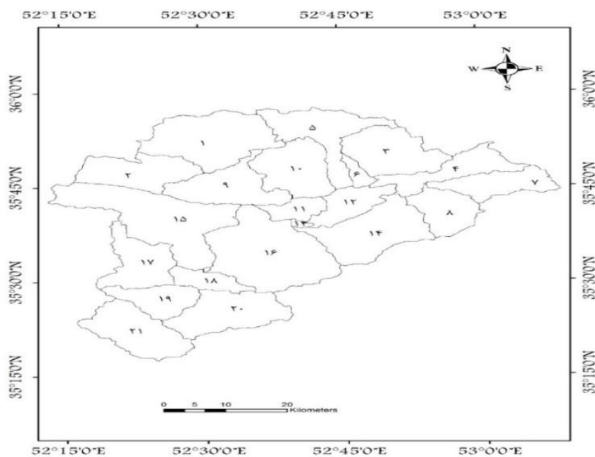
شکل ۲: نقشه زیرحوضه‌ها ترسیم شده در مدل سوات
