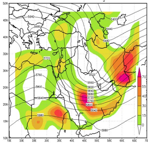
F: Convergence moisture 850 - 300 hPa و: همگرایی شار رطوبت
