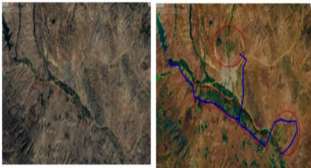
شکل ۳: عکس هوایی مسیر پایاب سد ستارخان اهر و مزارع و باغات ذینفع از این سد در سال ۲۰۱۸ و ۲۰۰۳ (منبع: تصاویر ماهواره‌ای گوگل ارث استان آذربایجان شرقی)
