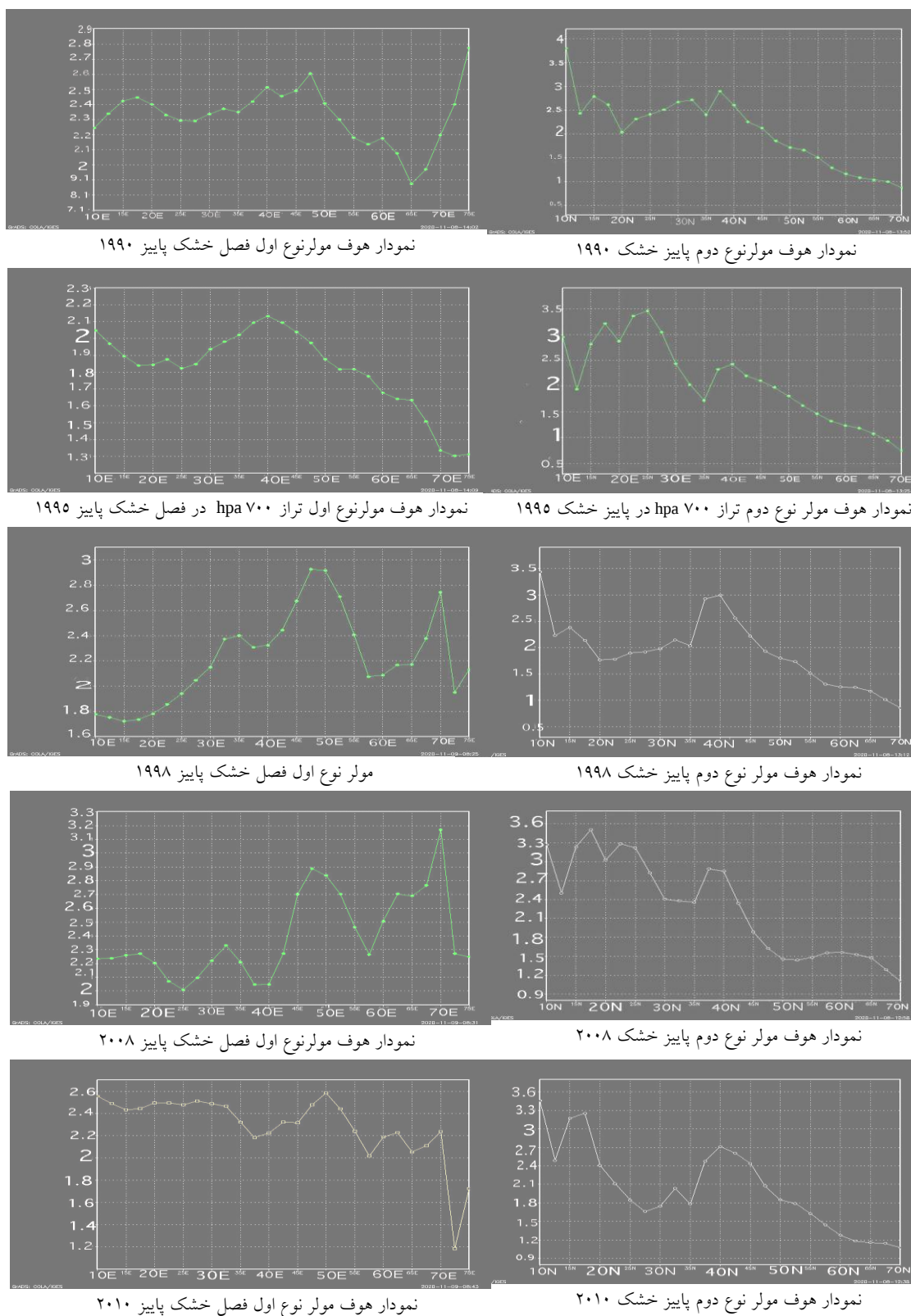
شکل ۳۰: نمودار هوف مولرنوع اول و دوم رطوبت ویژه تراز ۷۰۰ هکتوپاسکال فصول پاییز خشک سال‌های ۲۰۱۰، ۱۹۹۵، ۱۹۹۸، ۲۰۰۸ Figure 30: Hoff-Mueller diagram of the first and second types of specific humidity at 700 hpa in the dry autumn seasons of 2010, 2008, 1998, 1995, 1990
