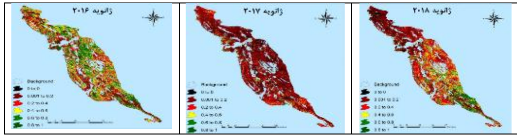
ادامه شکل ۲: شاخص VCI استان بوشهر (ژانویه ۲۰۰۱ تا ۲۰۱۸)
