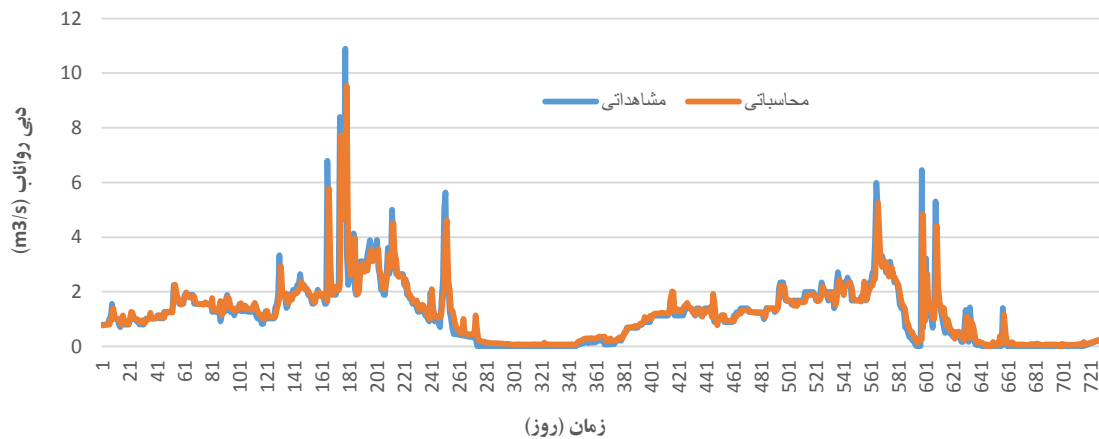
شکل ۷: نمودار سری زمانی دبی رواناب مشاهده‌ای و محاسباتی با مدل SVM در ایستگاه اورنگ برای دوره تست
