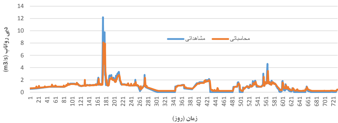
شکل ۸: نمودار سری زمانی دبی رواناب مشاهده‌ای و محاسباتی با مدل SVM در ایستگاه کاسین برای دوره تست
