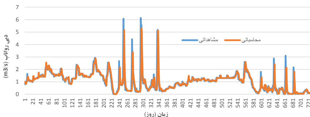
شکل ۹: نمودار سری زمانی دبی رواناب مشاهداتی و محاسباتی با مدل GEP در ایستگاه تازه‌کند برای دوره تست
