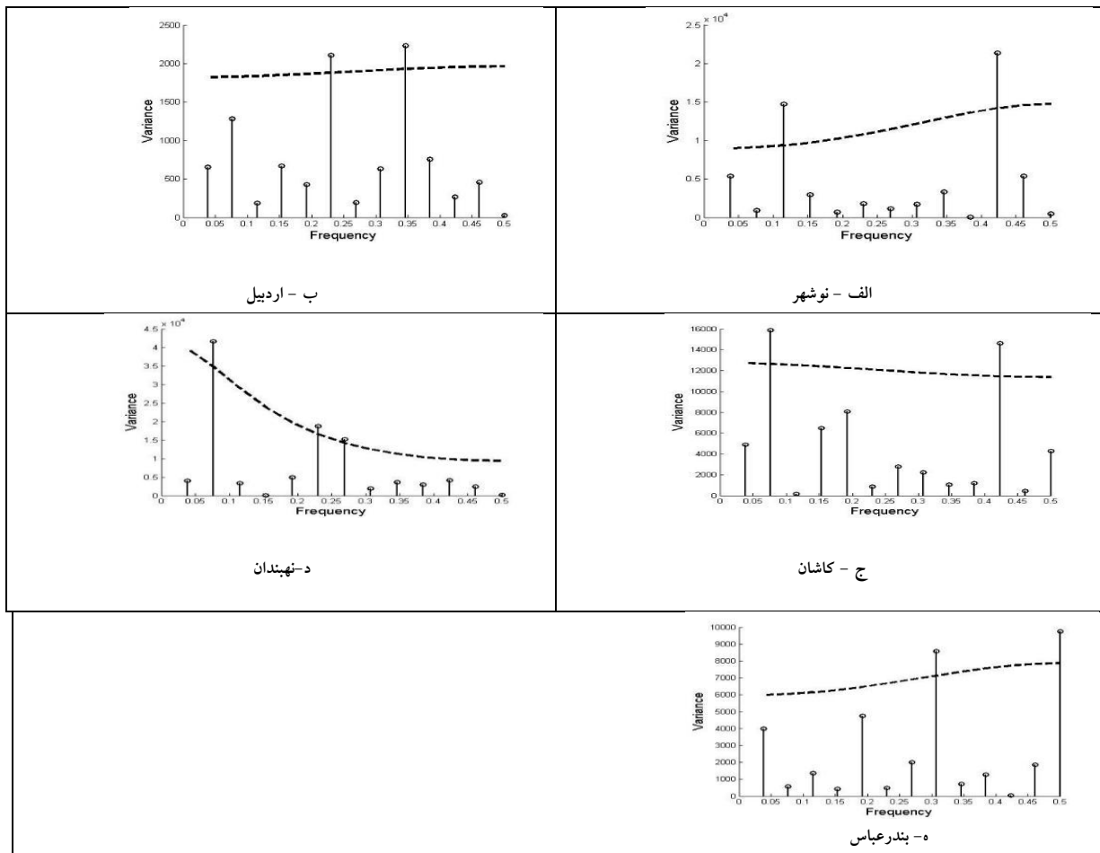
شکل ۲: دوره نگاره‌های چرخه‌های معنی‌دار (۹۵٪) ایستگاه‌های منتخب. الف) ناحیه ۱ بسیار دیرپا، ب) ناحیه ۲ دیرپا، ج) ناحیه ۳ میان‌دیرپا، د) ناحیه ۴ کوتاه، ه) ناحیه ۵ بسیار کوتاه فصل بارش کشور در دوره مرطوب (سپتامبر - می) سال‌های ۲۰۱۵-۱۹۹۰
