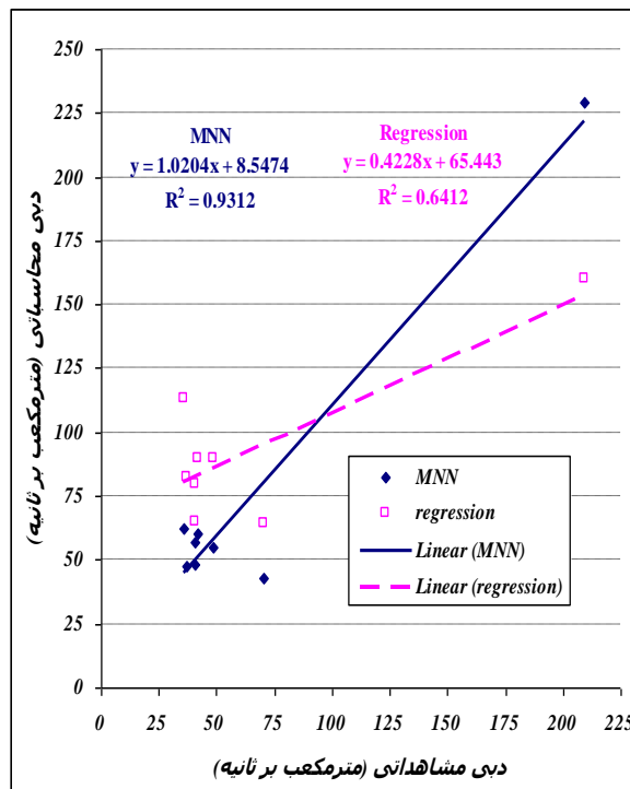
شکل شماره ۱۰- مقایسه مقادیر دبی مشاهده‌ای و محاسباتی حاصل از روندیابی هیدروگراف سیل با مدل های مختلف به ازای سیلاب فروردین ماه
