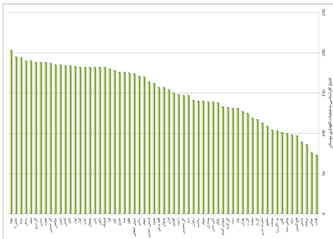
شکل ۹: رتبه‌بندی بوستان‌های منطقه ۱۷ بر اساس عملیات نگهداری بوستان Figure 9: Ranking the parks of region 17 based on park maintenance operations
