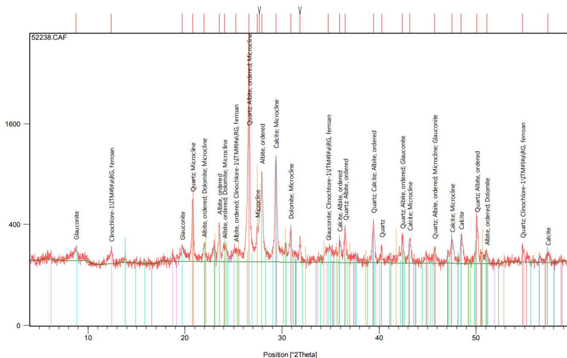
شکل ۸: نمودار طیف xrd کلوتک نمونه ۵
