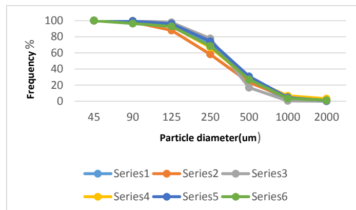
شکل ۸: نمایش منحنی های تجمعی رسوبات کوه ریگ در فواصل مختلف نیمرخ طولی
