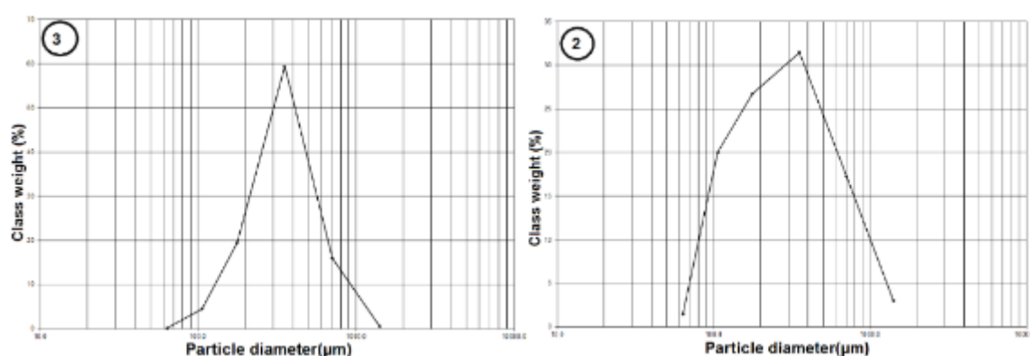
شکل ۷: نمایش منحنی توزیع پراکندگی رسوبات نمونه‌های ۲ و ۳ در امتداد نیمرخ طولی
