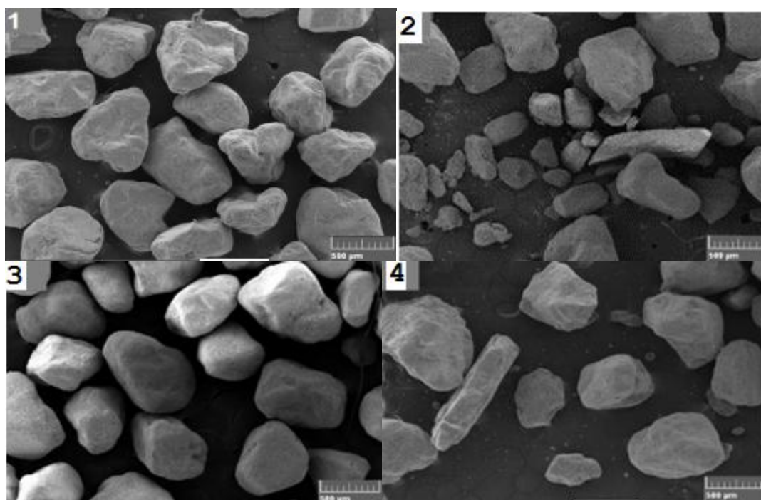
شکل ۱۲: نمایش تصویری از مورفوسکپی کانی های رسوبات کوه ریگ با بزرگنمایی ۶۰ و ۱۲۰ برابر با استفاده از میکروسکپ الکترونی روبشی
