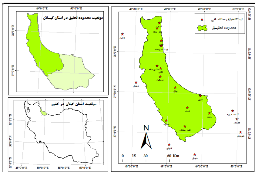
شکل ۱: موقعیت حوضه تالش- تالاب انزلی و ایستگاه‌های منتخب Figure 1: Location of Tالش Basin-Anzali lagoon and selected stations
