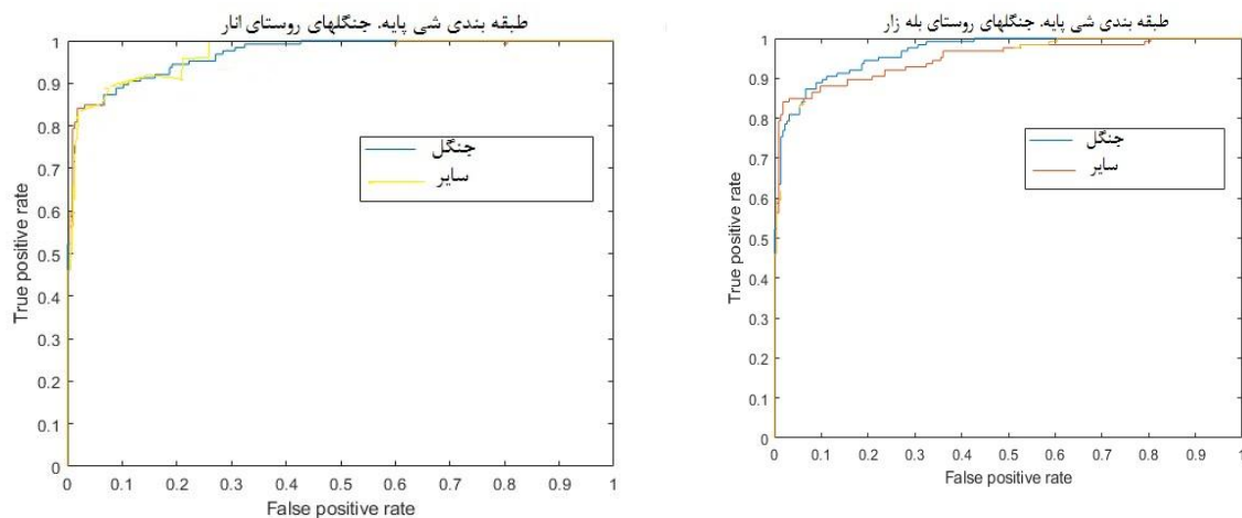
شکل ۱۰ الف: منحنی ROC طبقه‌بندی شی پایه. جنگل‌های روستای بله‌زار و انار به ترتیب از راست
