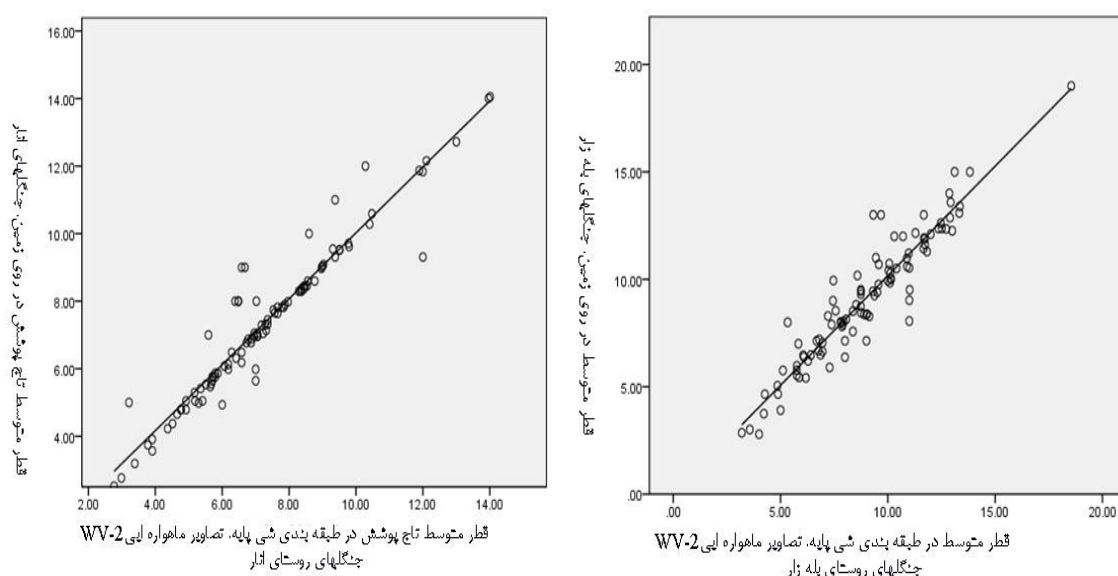
شکل ۸ ب: ارزیابی صحت قطر متوسط تاج پوشش در طبقه‌بندی شی پایه در تصاویر ماهواره‌ای WV-2 و روی زمین جنگل‌های روستای بهلهزار و انار به ترتیب از راست. به متر
