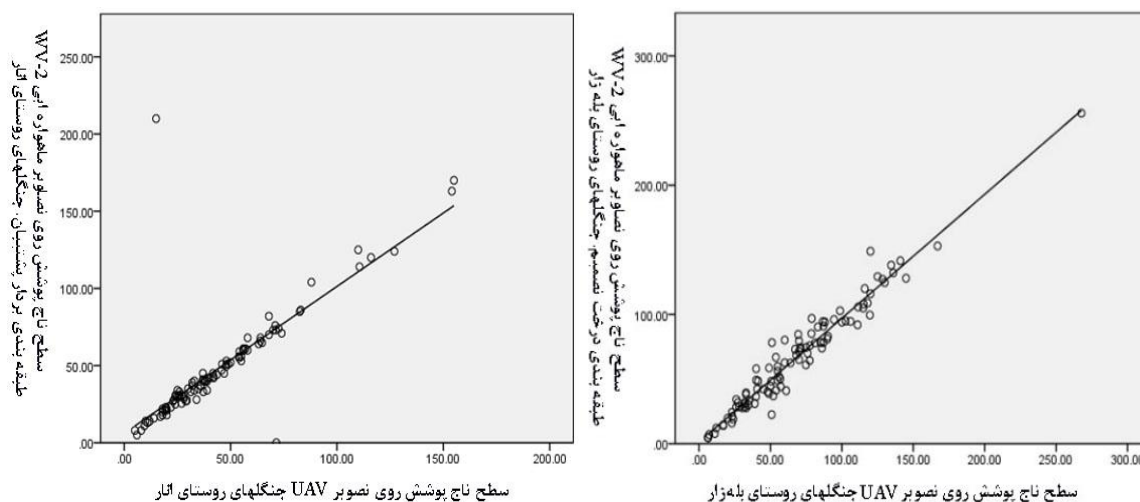
شکل ۷ الف: ارزیابی صحت سطح تاج پوشش در طبقه‌بندی بردار پشتیبان تصاویر ماهواره‌ای WV-2 و تصاویر UAV جنگل‌های روستای به‌زار و انار به ترتیب از راست. به مترمربع
