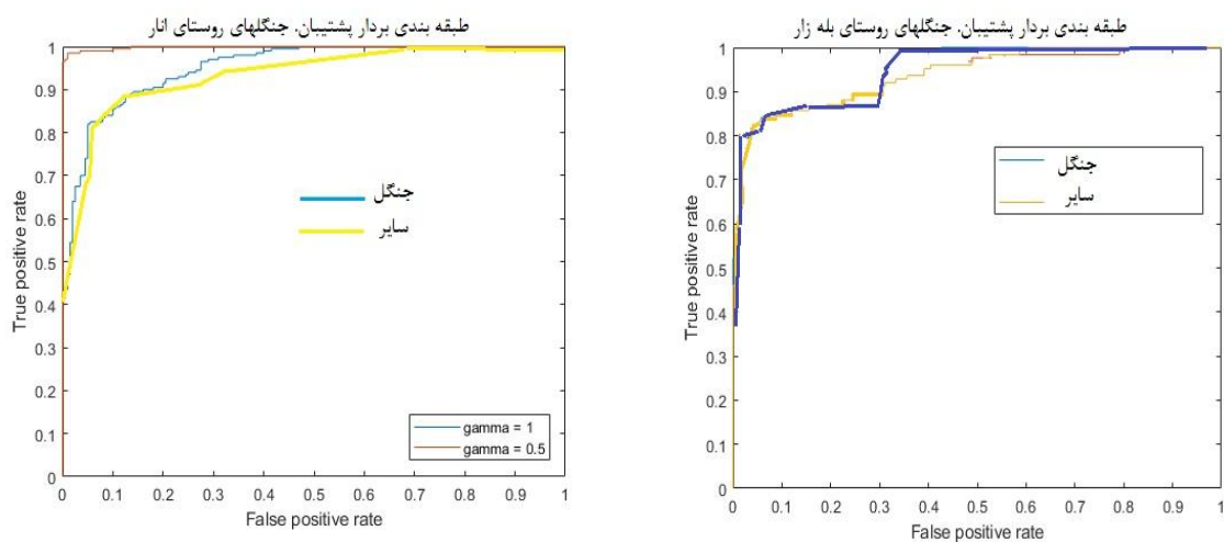
شکل ۱۰ ب: منحنی ROC طبقه‌بندی بردار پشتیبان. جنگل‌های روستای بله‌زار و انار به ترتیب از راست.
