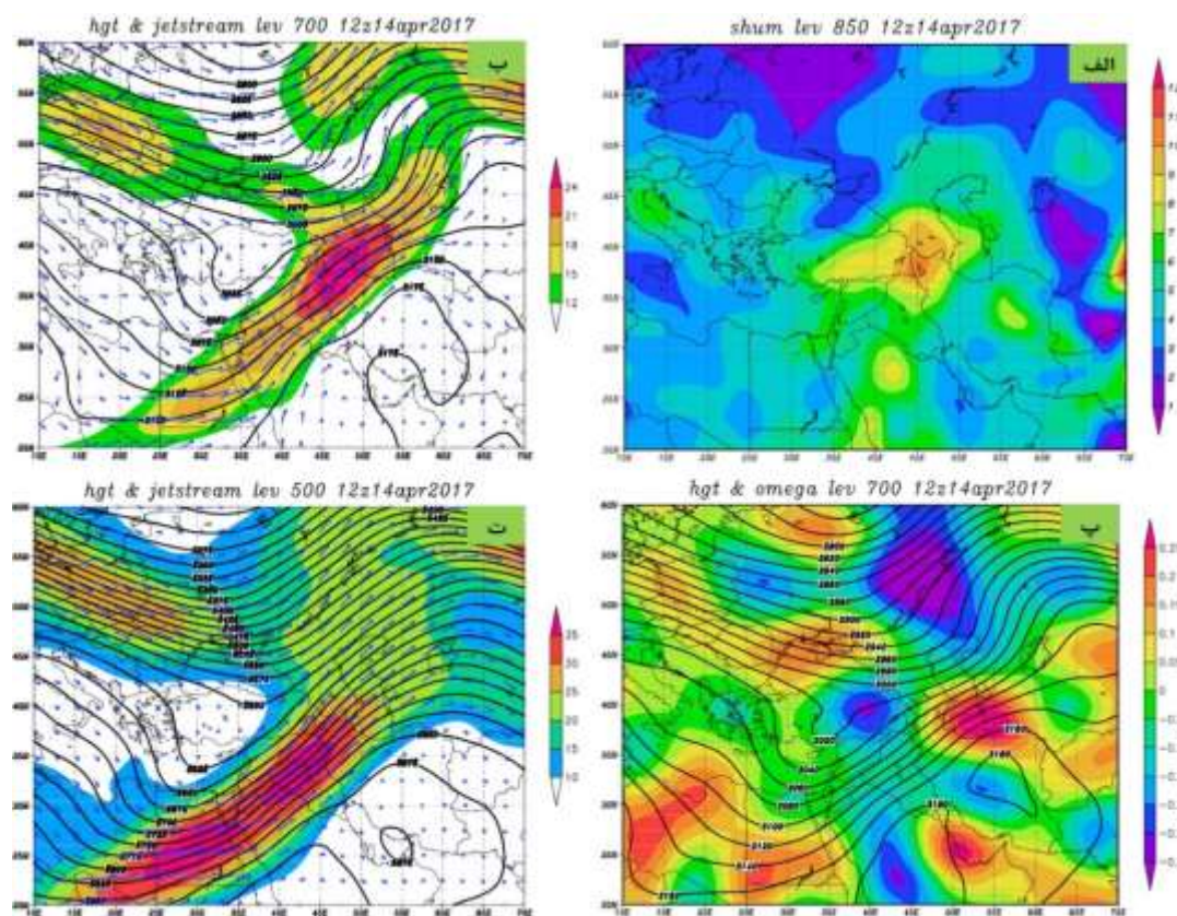
شکل ۵: نم و بزه در سطح ۸۵۰ میلی باری (الف) ارتفاع ژئوپتانسیل و رودباد در سطح ۷۰۰ میلی باری (ب)؛ ارتفاع ژئوپتانسیل و امگا در سطح ۷۰۰ میلی باری، (پ) و ارتفاع ژئوپتانسیل و رودباد در سطح ۵۰۰ میلی باری (ت) در روز ۱۴ آوریل ۲۰۱۷ ساعت ۱۲ z
