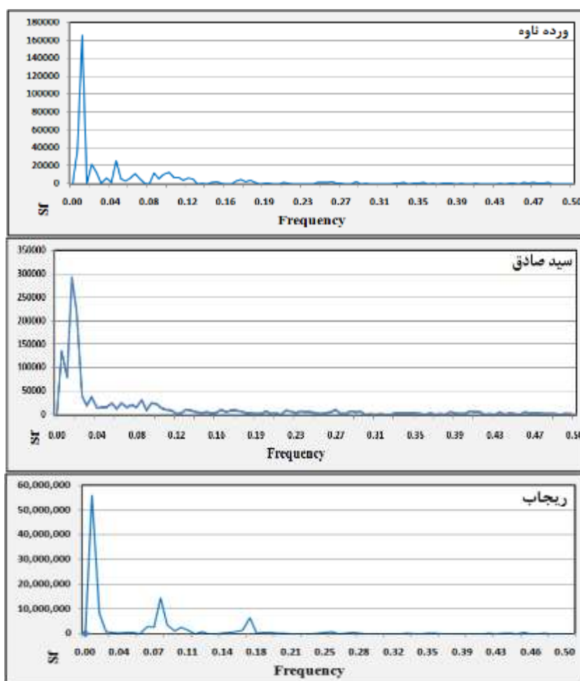
شکل ۷: تابع چگالی طیفی چشمه های ورده ناوه، سیدصادق، رجب، ماراب، قره بلاغ و چنارپیران
