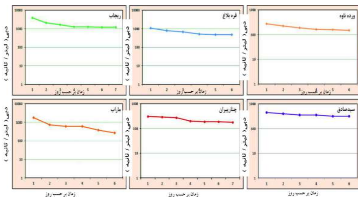
شکل ۳: منحنی فرود چشمه‌های شاخص توده دالاهو
