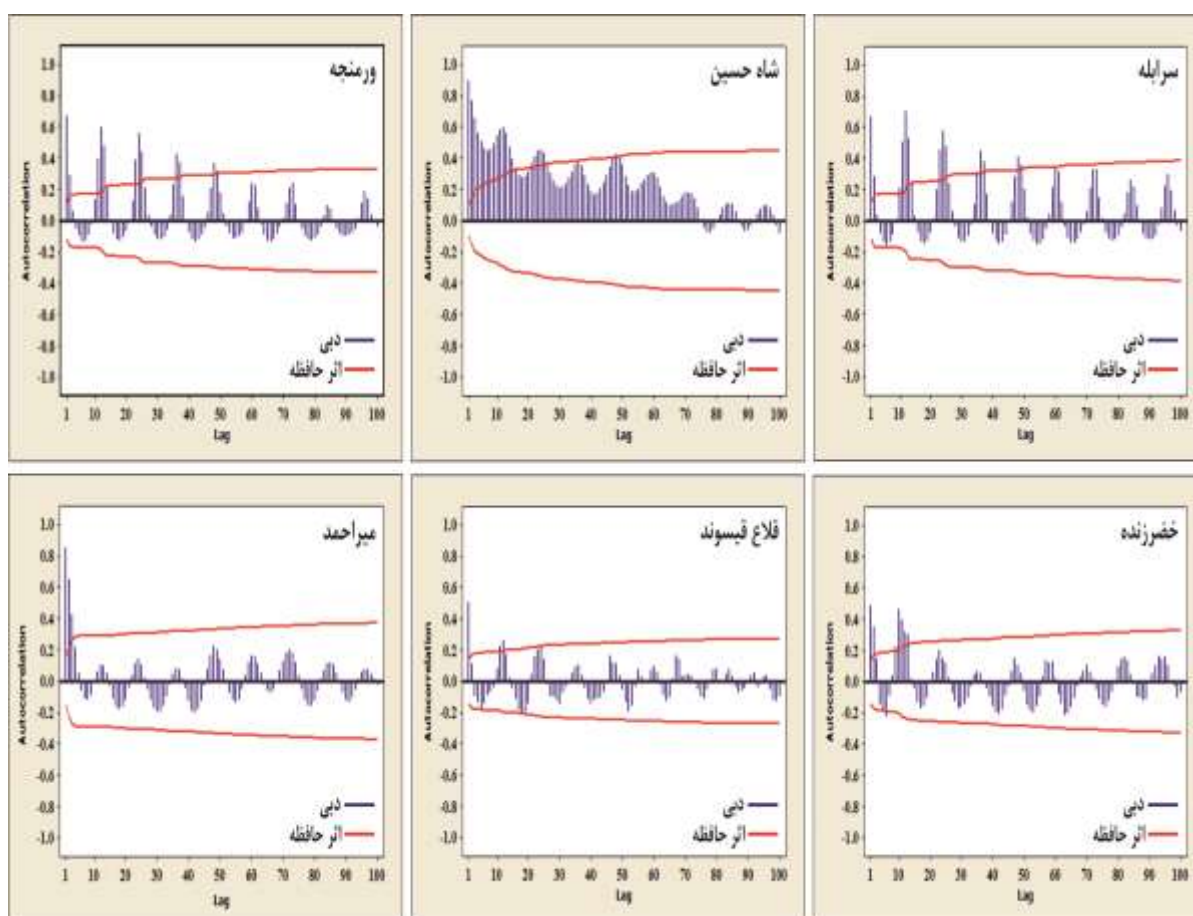
شکل ۶: کرولوگرام چشمه‌های ورم‌نجه، شاه‌حسین، سرابله، میراحمد، قلاع قیسوند و خضرزنده
