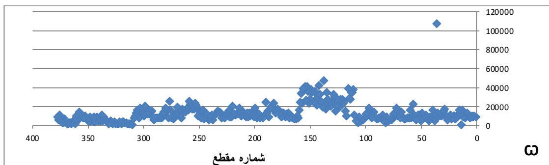
شکل ۱۴: میزان قدرت برش رودخانه ارس در مسیر جریان Figure 14: Cutting power of the Aras river in the flow direction
