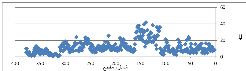
شکل ۱۳: میزان جریان رسوب در مسیر رودخانه ارس Figure 13: Sediment flow rate along the Aras River
