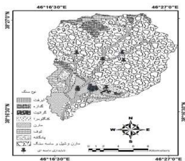
شکل ۲: نقشه‌ی زمین‌شناسی کمانج چای علیا
