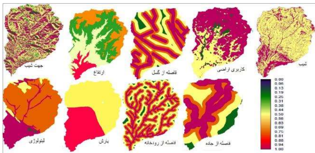
شکل ۴: فازی‌سازی لایه‌های موثر در وقوع ناپایداری دامنه
