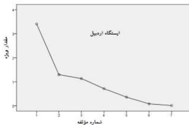
شکل ۳: نمودار واریزه‌ای (Scree Plot) در ایستگاه اردبیل
