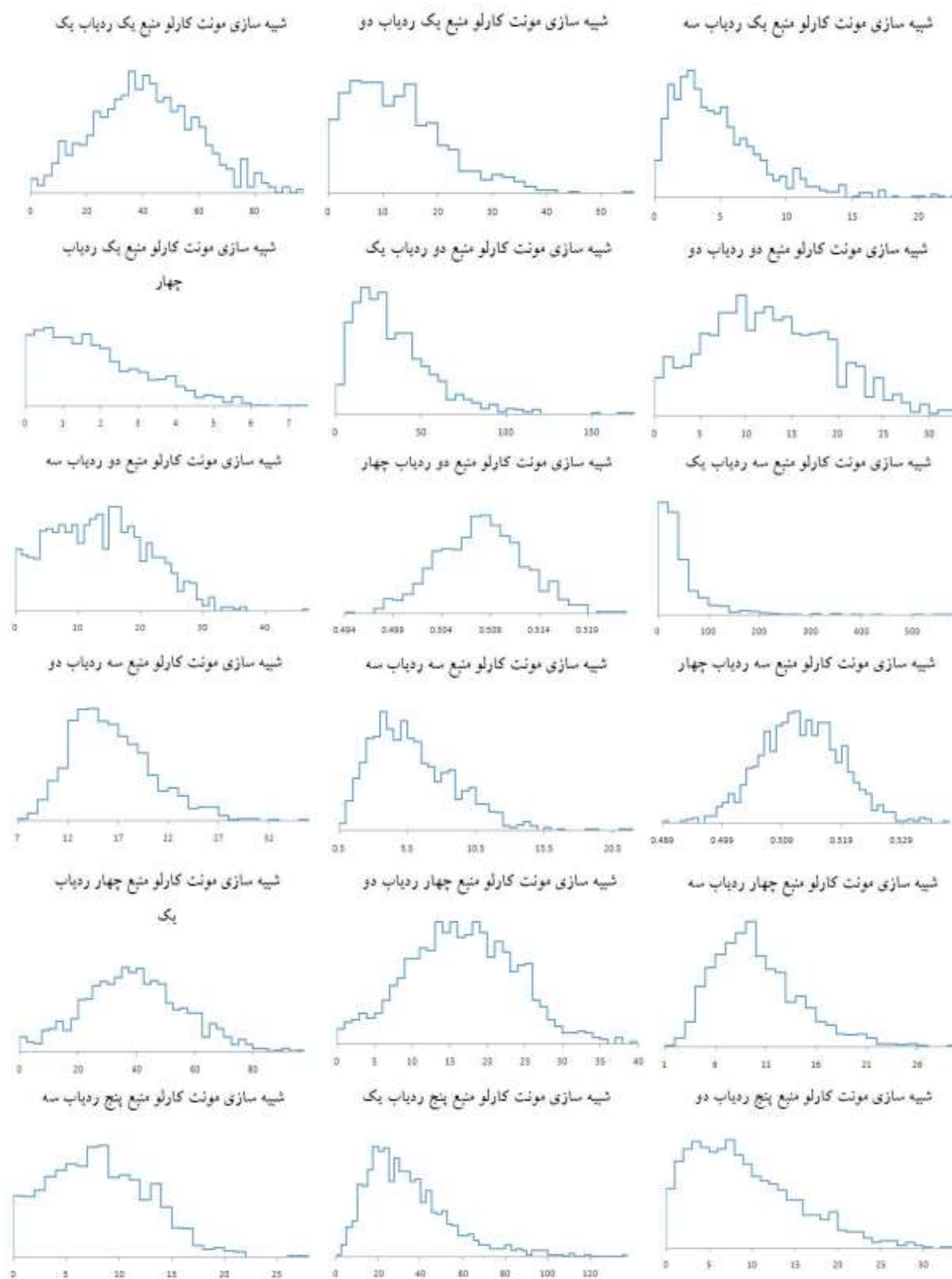
شکل ۵: برآورد مونٹ کارلو برای ردیاب‌های منابع مختلف سازندها
