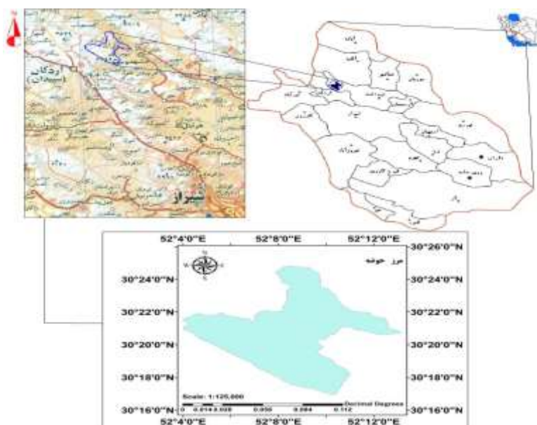
شکل ۱: موقعیت محدوده مورد مطالعه در استان فارس، ایران
