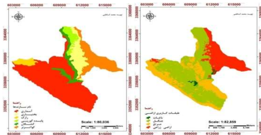
شکل ۲: نقشه واحدهای کاربری اراضی و سازندهای زمین‌شناسی به‌عنوان منابع مختلف تولیدکننده رسوب
