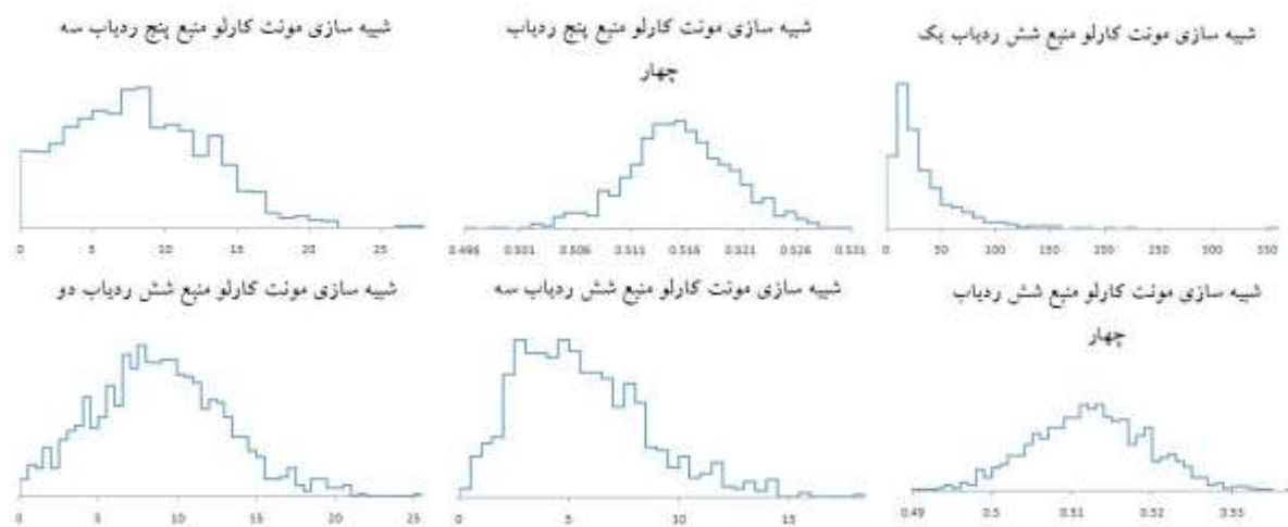
ادامه شکل ۵: برآورد مونٹ کارلو برای ردیاب‌های منابع مختلف سازندها
