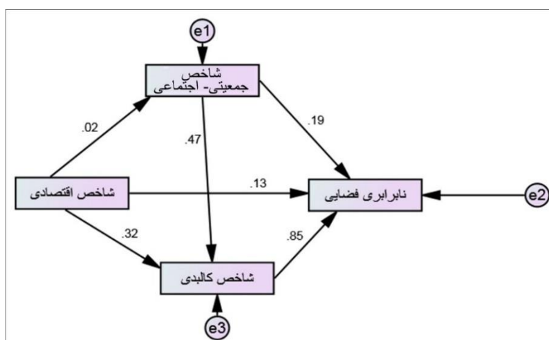
شکل ۳: نمودار مدل ساختاری پژوهش در حالت برآورد استاندارد
