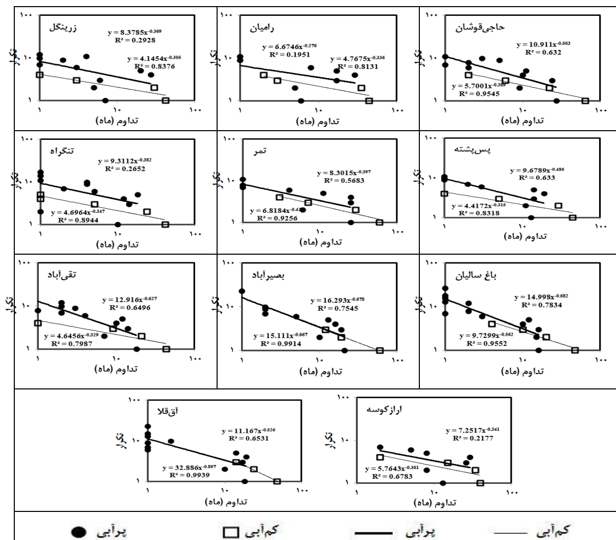
شکل ۳: پلات لگاریتمی دوگانه تعداد وقوع دوره‌های مختلف کم‌آبی و پرآبی در ایستگاه‌های هیدرومتری حوزه گرگانود
