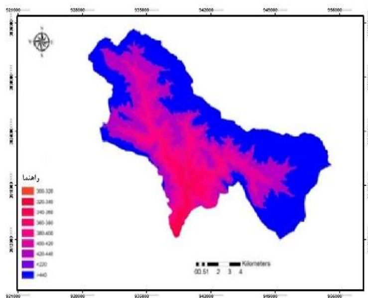
شکل ۳: نقشه منحنی بارش حوضه سامان (منبع: نقشه منحنی بارش حوضه مزلاغان)
