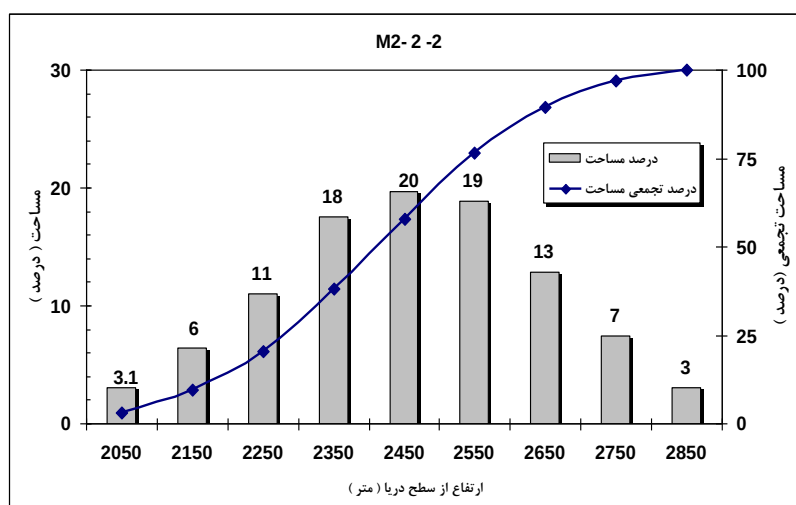
شکل ۲: نمودار توزیع سطح ارتفاع در زیر حوضه سامان
