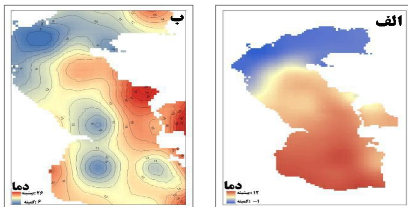
شکل ۱۲: الف) پهنه‌بندی دمای سطح آب برای روز قبل از بارش برف، ب) پهنه‌بندی تباین دمای هوای دومتري و دمای سطح آب برای روز همراه با بارش برف
