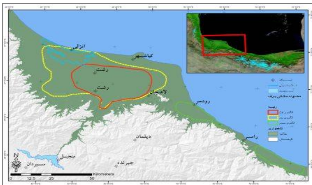
شکل ۱۶: الگوی مکانی برف‌های سنگین گیلان در کرانه جنوبی دریای خزر
