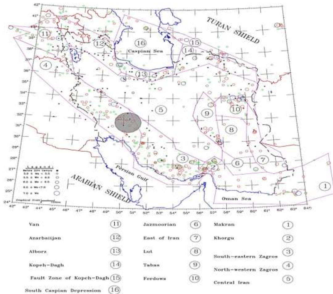
شکل ۳: موقعیت گستره مورد بررسی در نقشه ایالت های لرزه زمین ساختی ایران بر اساس مدل کمیته ملی سدهای بزرگ ایران (ICOLD, 1995)
