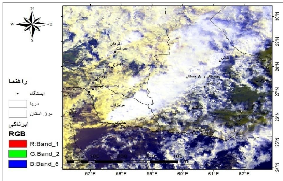
شکل ۳: ابرناکی آسمان در تاریخ ۲۳ ژانویه ۲۰۰۷ در ساعت UTC ۰۵:۹
