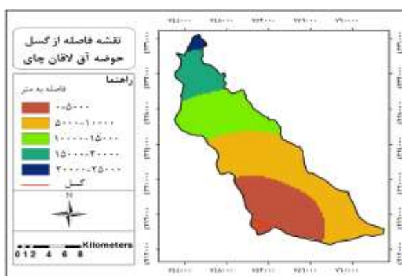
شکل ۴: نقشه فاصله از گسل
