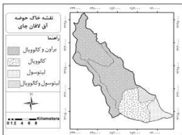
شکل ۱۱: نقشه خاک
