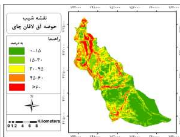
شکل ۶: نقشه شیب
