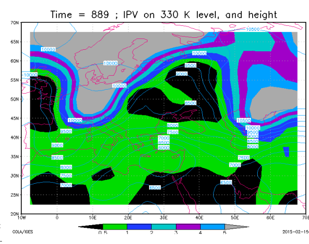
شکل ۱۹: تاوایی پتانسیلی ارتل در سطح همدمای ۳۳۰ کلوین
