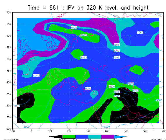
شکل ۲: تاوایی پتانسیلی ارتل در سطح همدمای ۳۲۰ کلون
