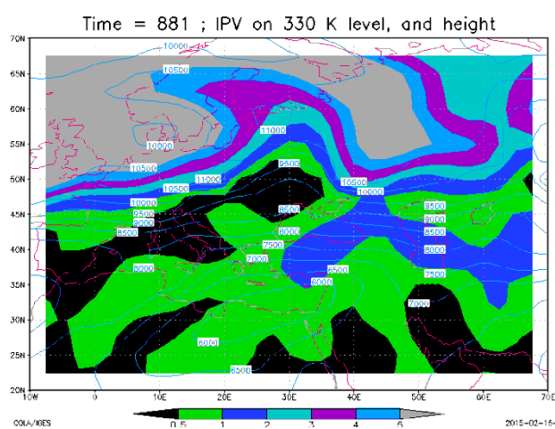
شکل ۱: تاوایی پتانسیلی ارتل در سطح همدمای ۳۳۰ کلون
