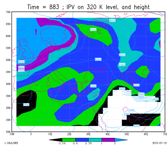
شکل ۴: تاوایی پتانسیلی ارتل در سطح همدمای ۳۲۰ کلون
