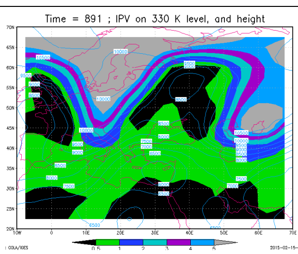
شکل ۲۱: تاوایی پتانسیلی ارتل در سطح همدمای ۳۳۰ کلین
