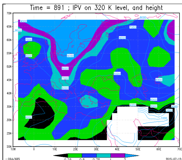
شکل ۲۲: تاوایی پتانسیلی ارتل در سطح همدمای ۳۲۰ کلین
