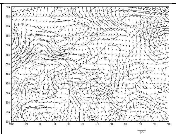
شکل ۲۳: الگوی گردشی تراز ۱۰۰۰ هکتوپاسکال ۲۰ مرداد (۱۳۸۰)
