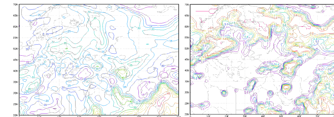
شکل ۱۶: همگرایی شار رطوبت تراز ۸۵۰ هکتوپاسکال ۱۹ مرداد ۱۳۸۰
