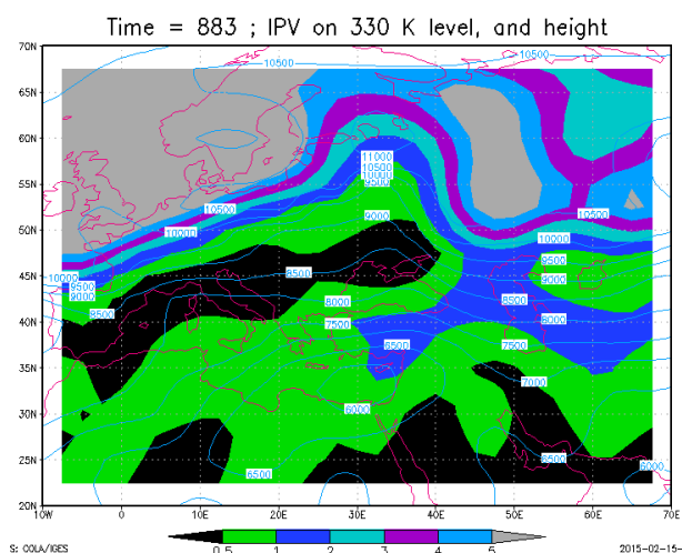
شکل ۳: تاوایی پتانسیلی ارتل در سطح همدمای ۳۳۰ کلون
