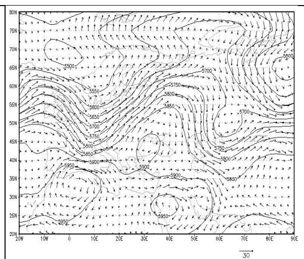
شکل ۲۵: الگوی گردشی تراز ۵۰۰ هکتوپاسکال ۲۰ مرداد ۱۳۸۰
