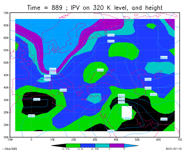
شکل ۲۰: تاوایی پتانسیلی ارتل در سطح همدمای ۳۲۰ کلونین
