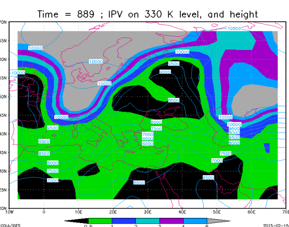
شکل ۱۹: تاوایی پتانسیلی ارتل در سطح همدمای ۳۳۰ کلونین
