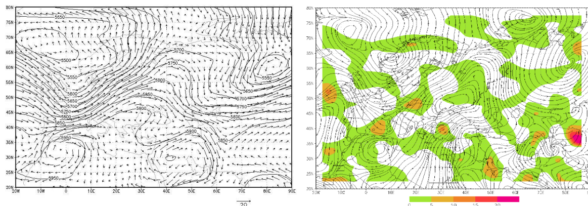
شکل ۱۵: الگوی گردشی تراز ۵۰۰ هکتوپاسکال ۱۹ مرداد ۱۳۸۰
