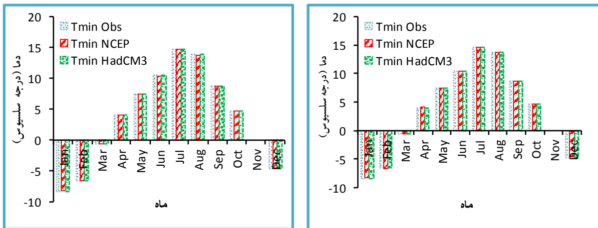
شکل ۲: مقادیر مشاهداتی و شبیه‌سازی شده دما در دوره ارزیابی مدل در ایستگاه سینوپتیک سقز
