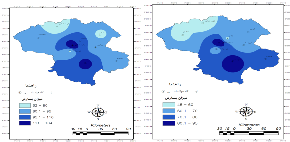
شکل ۹: توزیع جغرافیایی مقادیر بارش مرحله گل‌دهی
