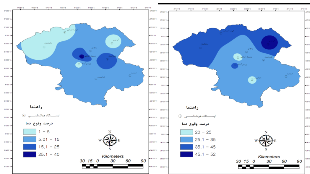
شکل ۱۵: توزیع جغرافیایی دماهای کم‌تر از ۹ درجه در پر شدن دانه
