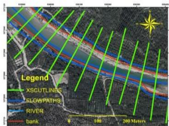
شکل ۱۰: نمایی از نقشه رقومی زمین و مقاطع عرضی
