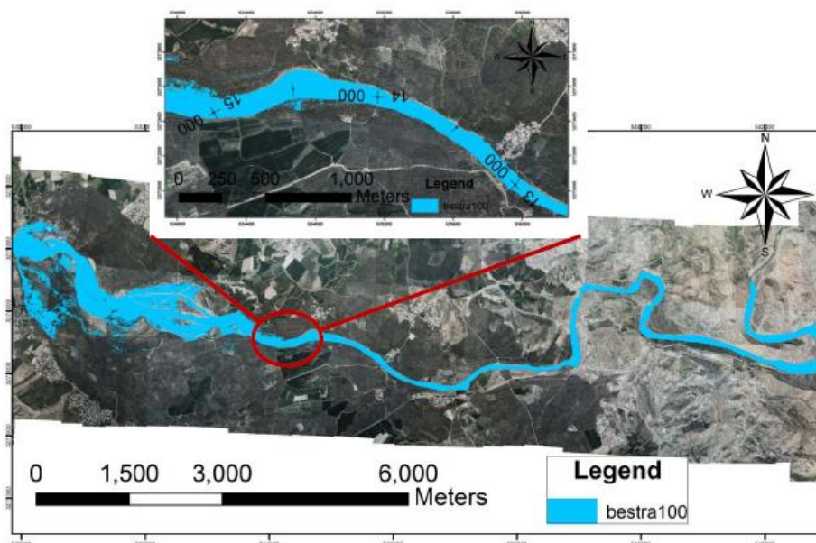
شکل ۱۸: پهنای سیلاب رودخانه‌ی شاپورخشت با دوره بازگشت ۱۰۰ سال
