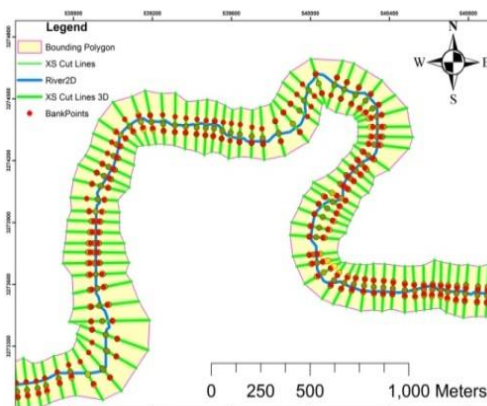
شکل ۱۱: نمای داده‌های ورودی به الحاقیه‌ی HEC-GeoRAS از نرم‌افزار HEC-RAS
