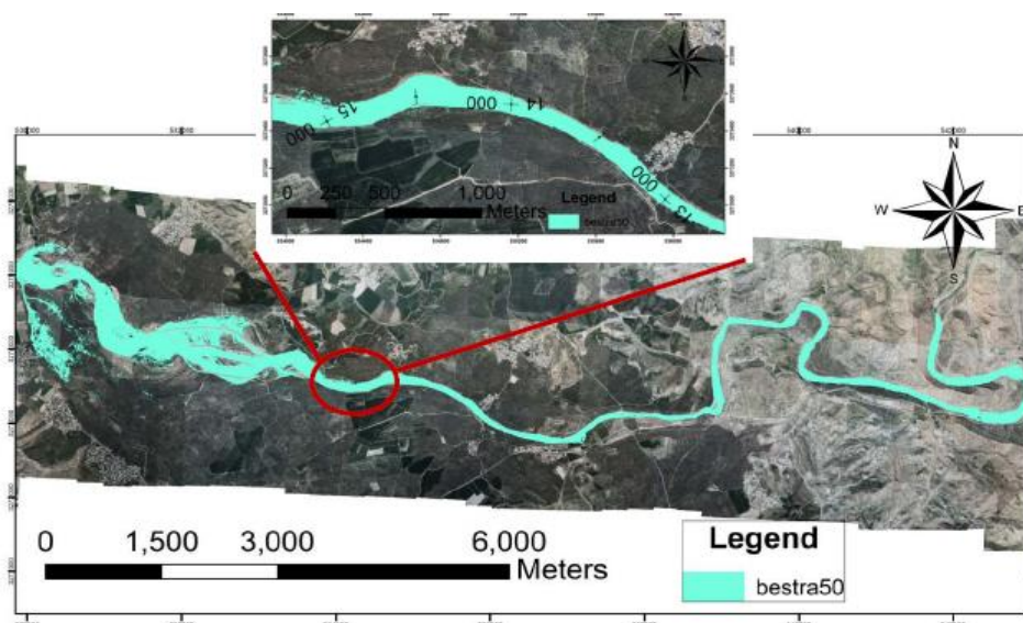
شکل ۱۷: پهنای سیلاب رودخانه‌ی شاپورخشت با دوره بازگشت ۵۰ سال
