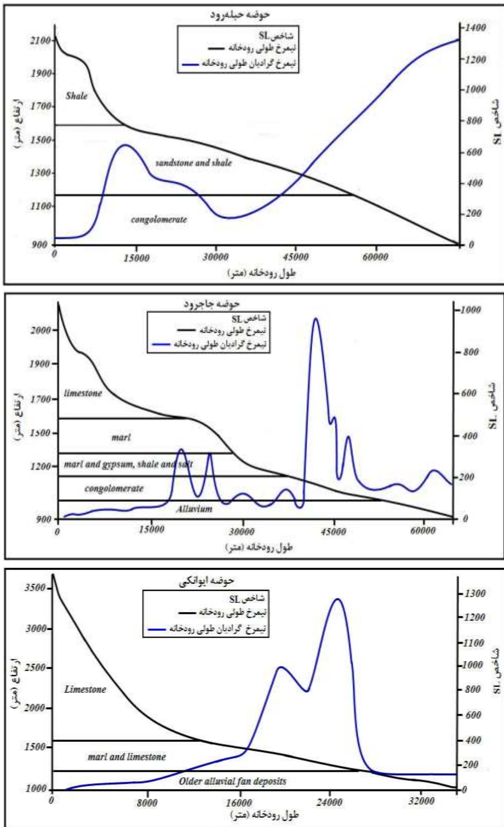
شکل ۸: نیمرخ وگرادیان طولی رودخانه‌های حبله‌رود، جاجرود و ابواتکی
