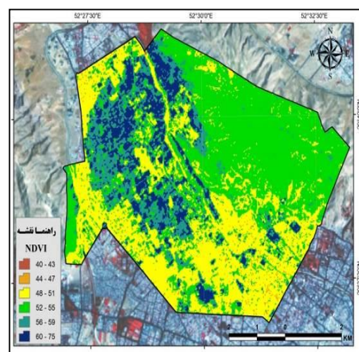
شکل ۳: نقشه درصد شاخص پوشش گیاهی در تاریخ: ۱۳۸۸/۱/۲
