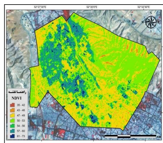
شکل ۱۵: نقشه درصد شاخص پوشش گیاهی در تاریخ: ۱۳۸۹/۱۰/۱
