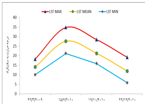
شکل ۲۰: روند کمینه، میانگین و بیشینه دمای سطح زمین در تاریخ‌های چهارگانه
