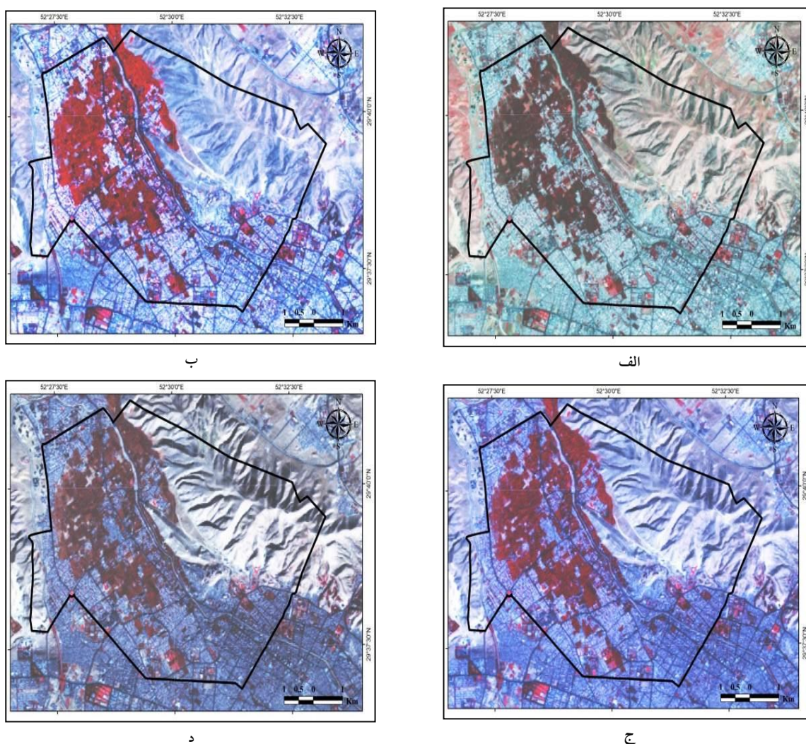
شکل ۲: ترکیب کاذب رنگی (RGB ۴۳۲) تصویر ماهواره‌ای منطقه یک شهر شیراز در تاریخ‌های
