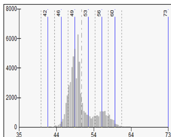
شکل ۱۷: انحراف معیار درصد شاخص پوشش گیاهی در تاریخ: ۱۳۸۹/۱۰/۱ شکل ۱۸: انحراف معیار دمای سطح زمین در تاریخ: ۱۳۸۹/۱۰/۱
