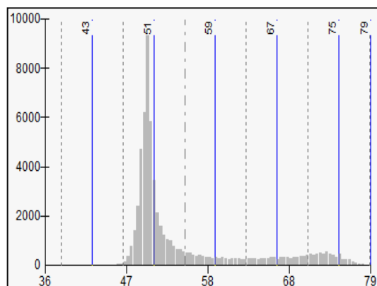
شکل ۹: انحراف معیار درصد شاخص پوشش گیاهی در تاریخ: ۱۳۸۹/۴/۲۴
