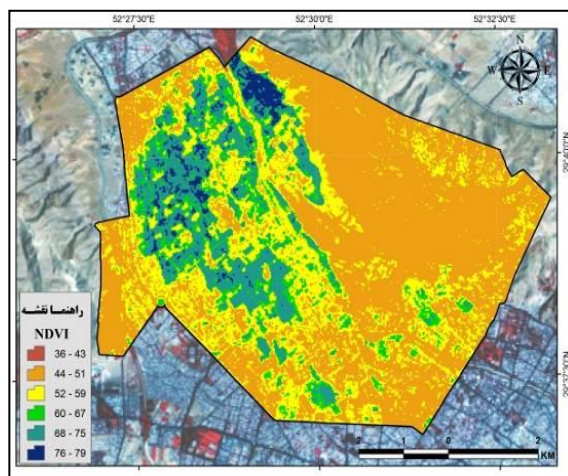
شکل ۷: نقشه درصد شاخص پوشش گیاهی در تاریخ: ۱۳۸۹/۴/۲۴
