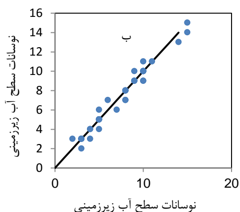
شکل ۷: نمودار حاصل از مقادیر بهینه مدل شبکه بیزین برای داده‌های ثبت شده مرحله صحت سنجی (الف) مقادیر محاسباتی و مشاهداتی نسبت به زمان (ب) نمودار پراکنش میان مقادیر مشاهداتی و محاسباتی
