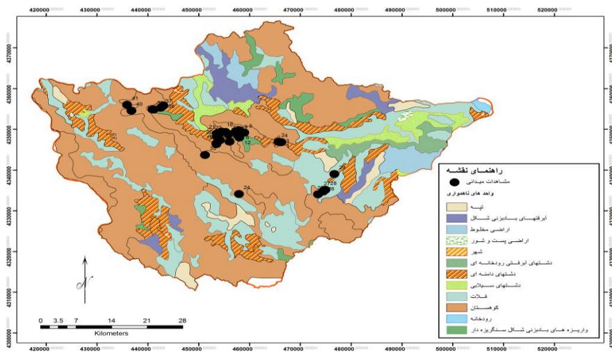
شکل ۵: واحدهای ناهمبوری و نقاط برداشت در حوضه زنگمار
