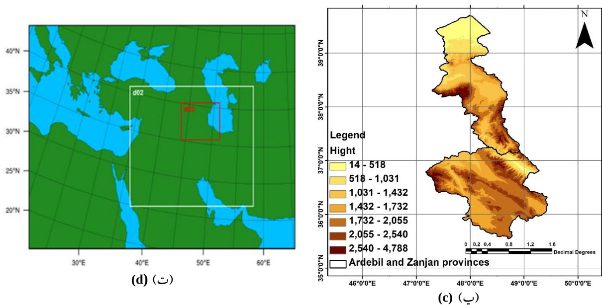
شکل ۱: الف و ب) موقعیت جغرافیایی استان های اردبیل و زنجان و ایستگاه های سینوپتیک آن ها که برای ارزیابی شبیه سازی مدل WRF استفاده شدند. پ) مدل رقومی ارتفاع استان های زنجان و اردبیل به واحد متر ( https://girs.ir ). ت) شبکه های محاسباتی مدل WRF.
