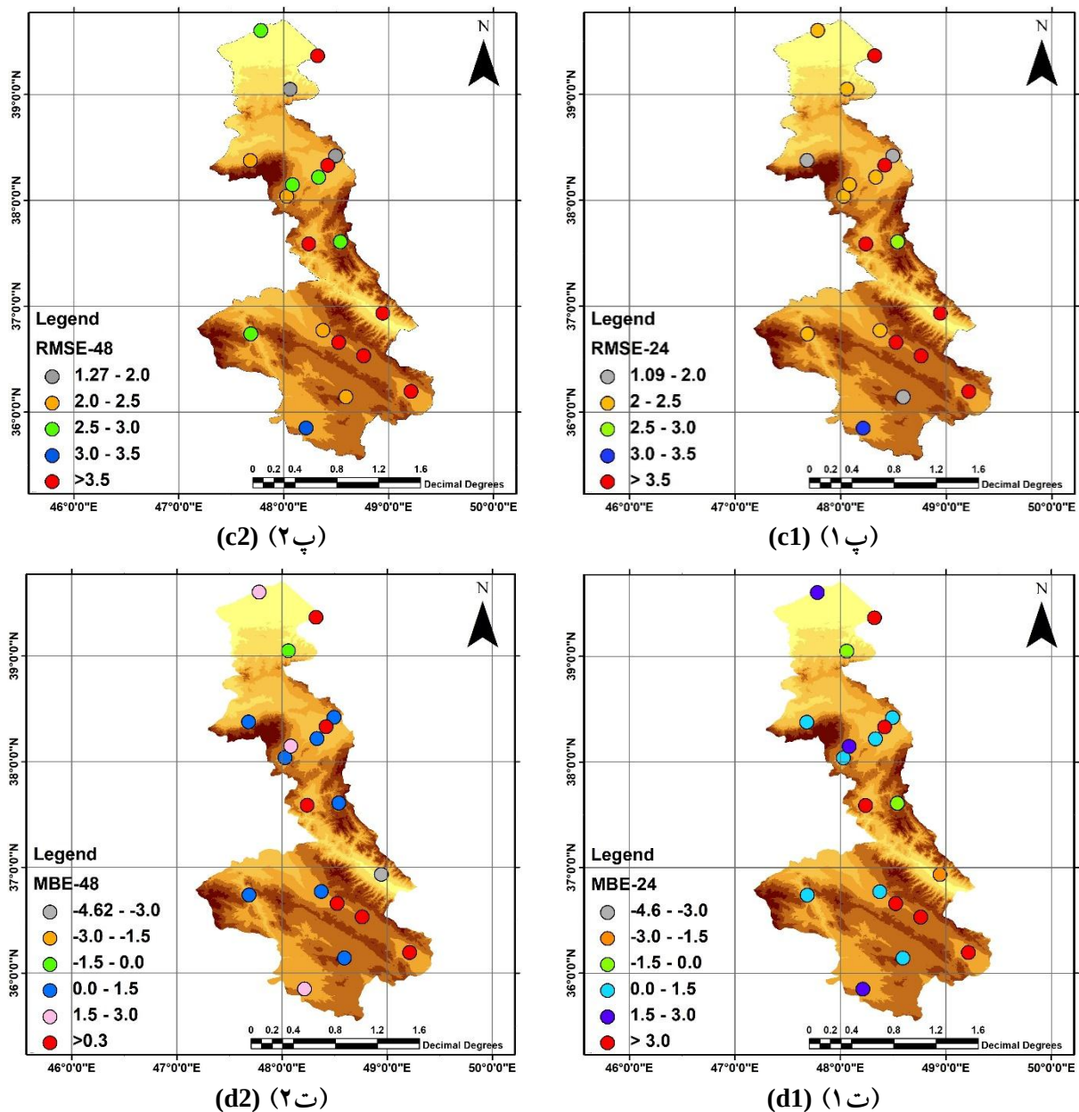
شکل ۵: نقشه های توزیع جغرافیایی شاخص های محاسبه شده در ارزیابی شبیه سازی های ۲۴ و ۴۸ ساعته مدل WRF: الف ۱، ۲) R
