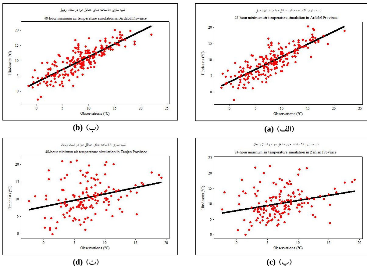
شکل ۲: نمودارهای پراکندگی داده های دمای حداقل مشاهده شده در برابر داده های پیش یابی شده مدل WRF برای شبیه سازی های ۲۴ و ۴۸ ساعته در (الف و ب) استان اردبیل؛ (پ و ت) استان زنجان.
