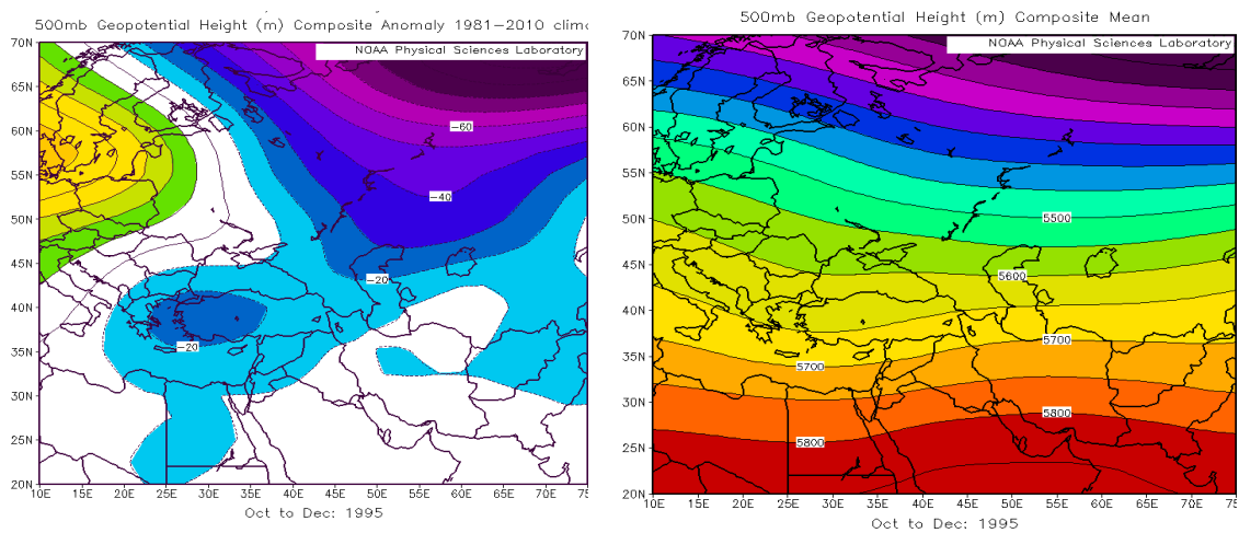
شکل ۸: نقشه تراز ۵۰۰ هکتوپاسکال و شکل ۹: نقشه ناهنجاری تراز ۵۰۰ فصل خشک پاییز ۱۹۹۵ Figure 8: 500 hPa level map and Figure 9: level 500 anomaly map of the dry season Autumn 1995
