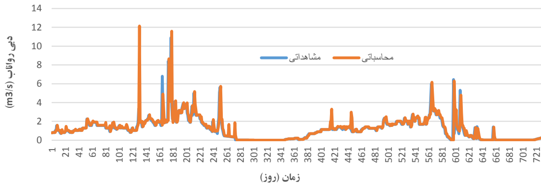
شکل ۱۳: نمودار سری زمانی دبی رواناب مشاهده‌ای و محاسباتی با مدل GEP در ایستگاه اورنگ برای دوره تست
