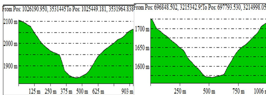
شکل ۳: نیم‌رخ عرضی: سمت راست کانیون و سمت چپ تنگ؛ استخراج از Global Mapper.
