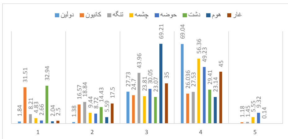
شکل ۱۰: نمودار پراکندگی عوارض کارستی در طبقات دمایی-بارشی در زمان کنونی.
