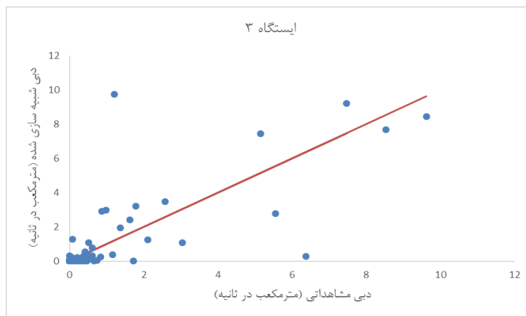
شکل ۶: دبی‌های مشاهداتی و شبیه‌سازی شده برای دوره صحت‌سنجی در ایستگاه سه Figure 6: Observed and simulated flow in validation period in Station 3
