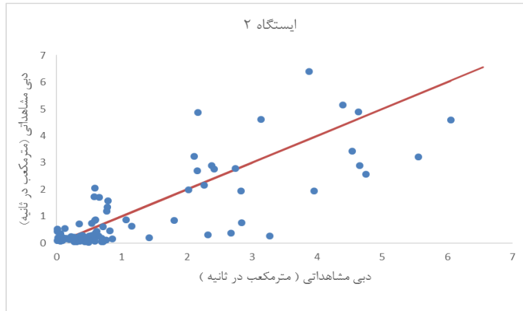
شکل ۵: دبی‌های مشاهداتی و شبیه‌سازی شده برای دوره صحت‌سنجی در ایستگاه دو Figure 5: Observed and simulated flow in validation period in Station 2
