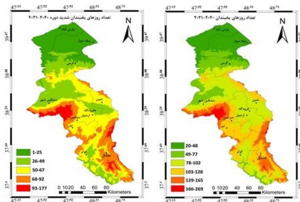
شکل ۴: نقشه پهنه بندی متوسط تعداد روزهای یخبندان: تعداد کل روزهای یخبندان (راست) تعداد روزهای یخبندان شدید (چپ) (۲۰۲۱-۲۰۴۰) Figure 4: Spatial distribution map of mean number of frost days: total frost day (right) severe frost day (left) (2021-2040)
